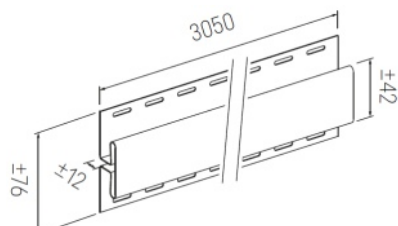
SV-18 spojovací profil "H"
