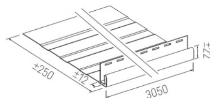
SV-19 římsový profil
