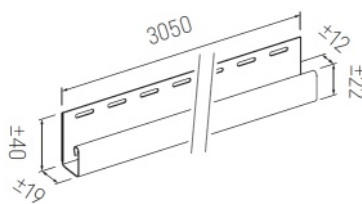
SV-15 ukončovací profil "J"
