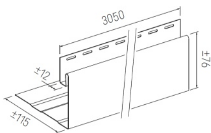
SV-17 okenní špaletový profil
