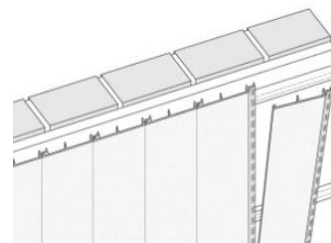
vinyTherm se montuje svisle i vodorovně
