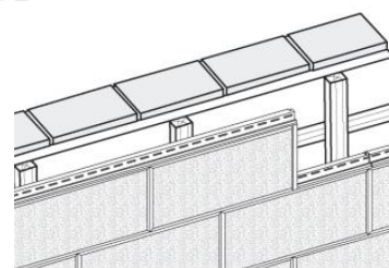
desky vinyStone se montují vodorovně
